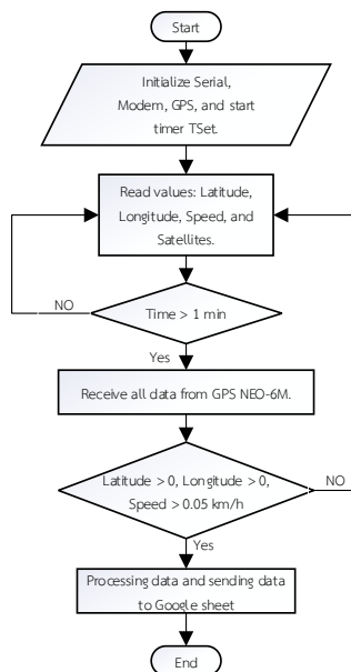
รูปที่ 3 แสดงการทำงานของอุปกรณ์ต้นแบบติดตามและบันทึกข้อมูลวัวด้วย GPS และ IoT
