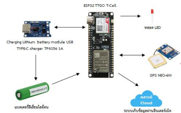
รูปที่ 1 แสดงโครงสร้างอุปกรณ์ต้นแบบติดตามและบันทึกข้อมูลด้วย GPS และ IoT
