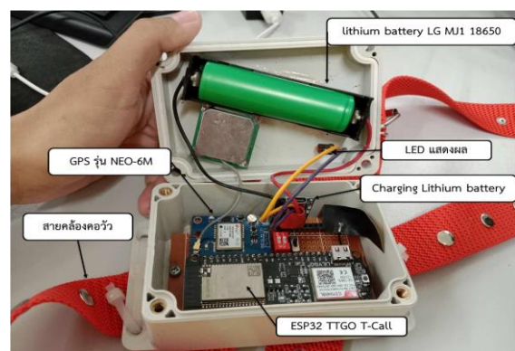
รูปที่ 2 แสดงวงจรและอุปกรณ์ทั้งหมดบรรจุในกล่อง
